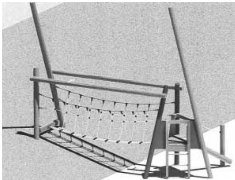
Einstieg mit Hängebrücke
