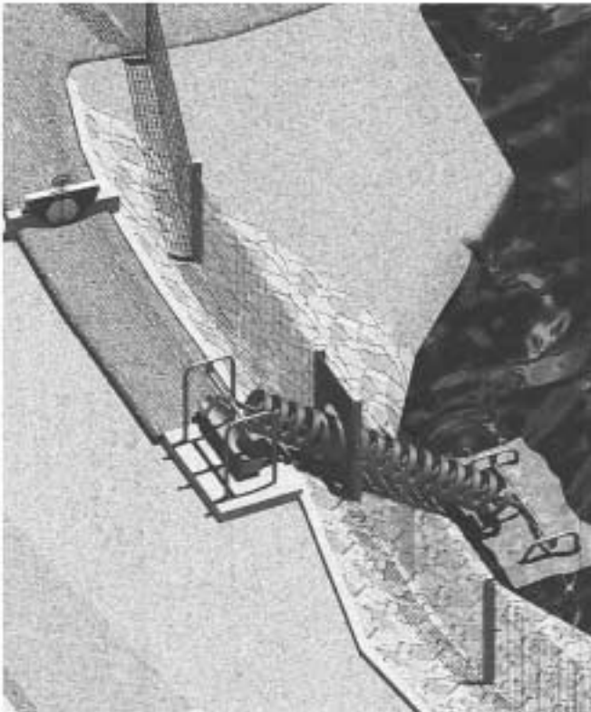
Vils-Brunnen Archimedische Spirale mit Stauklappe und barrierefreiem Zugang
